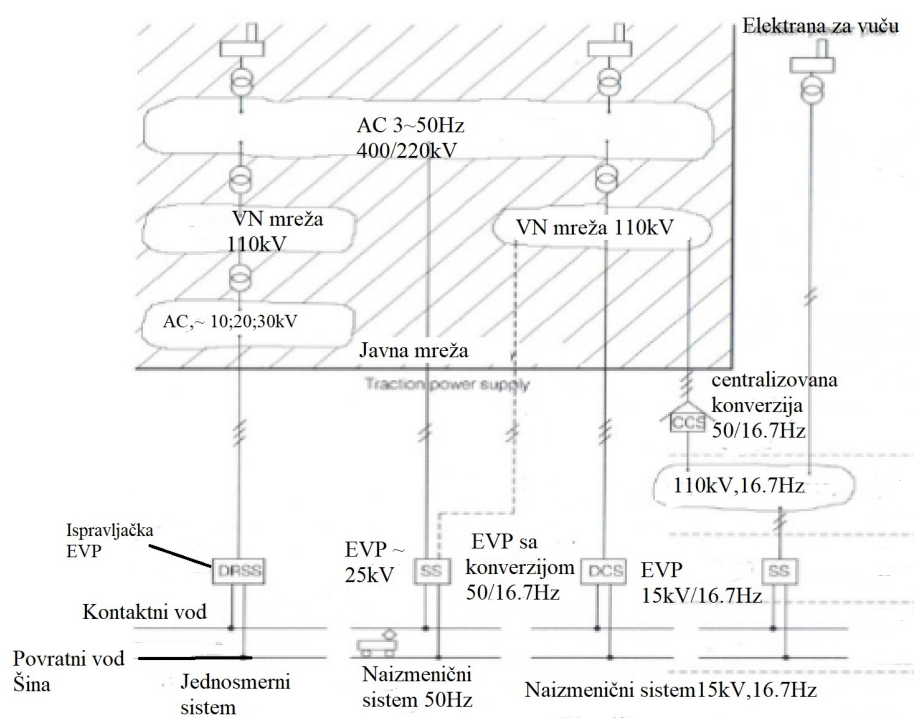
Slika 2: Elektroenergetski sistemi za železnicu
