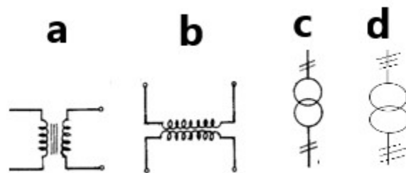
Slika 4: Simboli za šematsko prikazivanje transformatora
