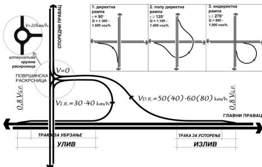
Слика 4-05: Меродавне брзине и капацитети за пројектовање појединачних елемената денивелисаних раскрсница.
