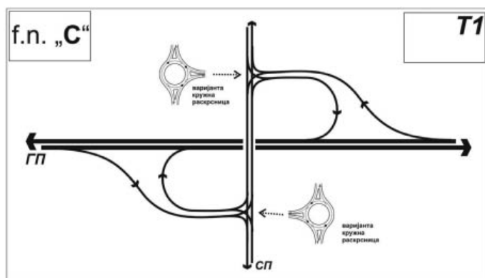
Слика 4-11: Денивелисана раскрсница облика "ПОЛА ДЕТЕЛИНЕ".
