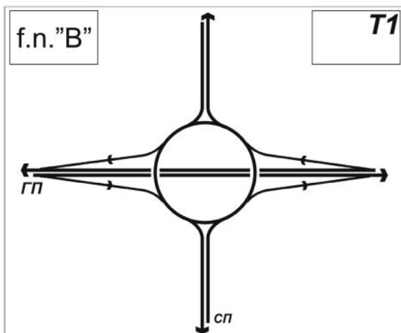
Слика: 4-12: Денивелисана раскрсница "КРУЖНИ ПОДЕОНИК".
