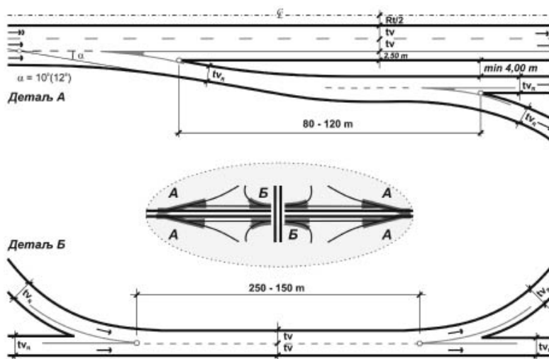
Слика 5-10: Типска решења рачвања и преплитања једносмерних рампи.
